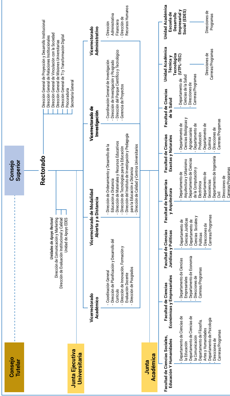
Figura 1. Estructura Académica
